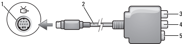
1 S-video TV-out-aansluiting 2 composietvideo-aansluiting 3 S/PDIF digitale audioaansluiting 4 composietvideo-uitvoeraansluiting 5 S-video-aansluiting
